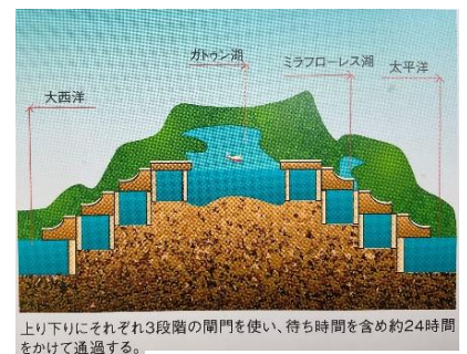
パナマ運河の構造
